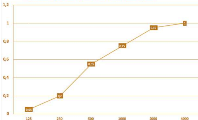
Schallabsorptionswerte SilentFiber TORF Akustikplatte
