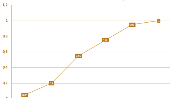
Schallabsorptionswerte SilentFiber TORF Akustikplatte
