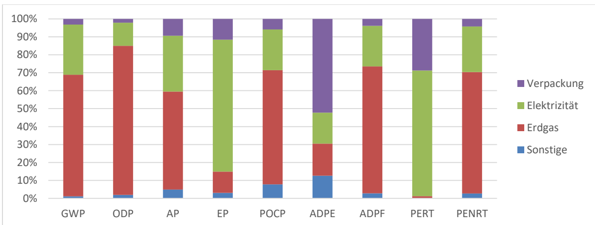
Abbildung 3-5: Die Verursacher der Belastungen an der Herstellung (A3) der Heradesign-Platten pro Quadratmeter
